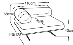
1-element armrest left incl. 1 MBA Item number: D153106
